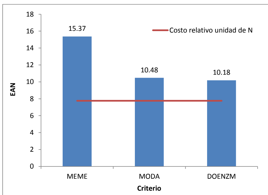
Figura 23. Eficiencia agronómica del nitrógeno aplicado y relación con margen bruto y costo relativo de la unidad de nitrógeno.
