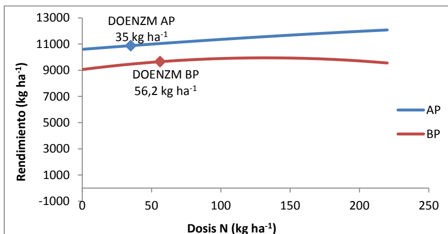
Figura 22. Rendimiento de maíz ( \text{kg ha}^{-1} ) en función de la dosis de N ( \text{kg ha}^{-1} ) sitio Las Vertientes, Campaña 2012-13. Línea azul AP (alta producción), línea roja BP (baja producción).
