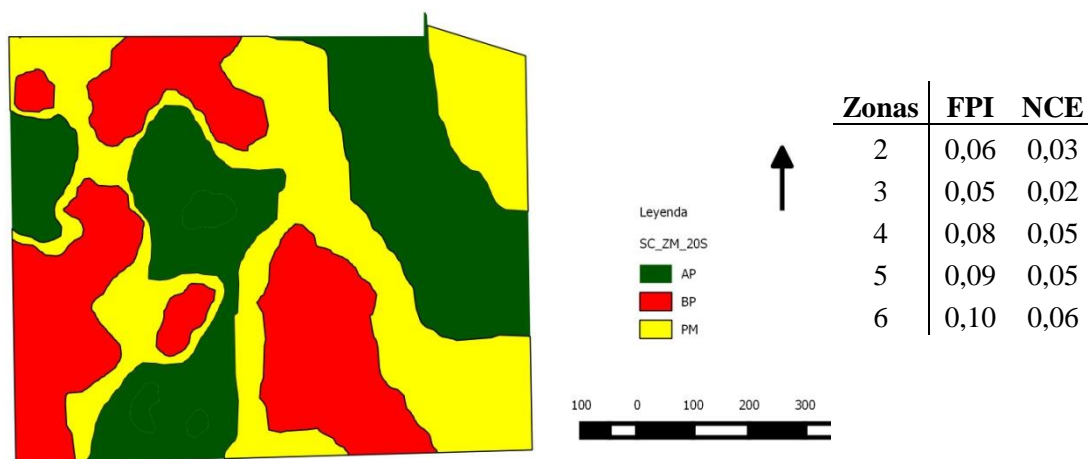
Figura 2. Zonas de manejo Santa Clara (Córdoba). AP: alta producción (verde), BP (baja producción) PM (Producción Media). Valores de FPI (índice de borrosidad) y NCE (índice de entropía) por cantidad de zonas.
