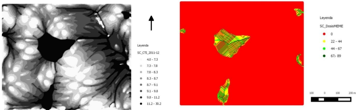
Figura 9. Mapa de CTI, (izquierda), mapa de prescripción de N en base a MEME año seco (derecha), sitio Santa Clara, Córdoba.
