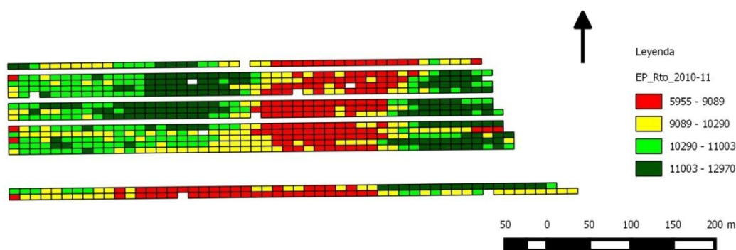
Figura 7. Mapa de rendimiento del ensayo, El Piquete Córdoba.
