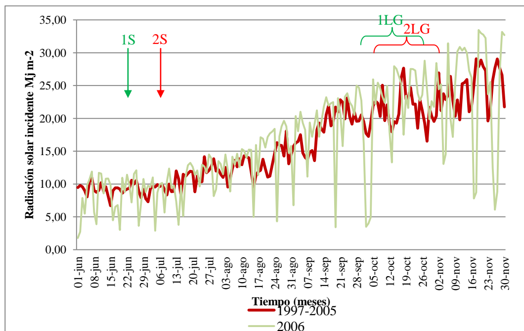
Figura 3. Radiación solar para el periodo Junio 2006 a Noviembre 2006 (siembra a cosecha). La línea verde representa la radiación solar para el ciclo del cultivo durante el año del ensayo y la línea roja, la radiación solar media para el período 1997-2005.
